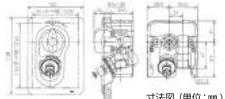
寸法図 (単位: mm)
