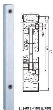
HI塩ビ管配管
