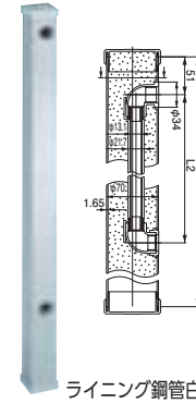
ライニング鋼管白管
